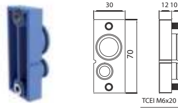
M221-S Tapón terminal izquierdo
