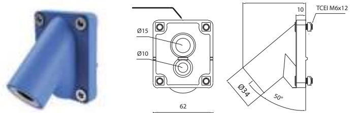
M231-012045 Toma inclinada 1/2"
