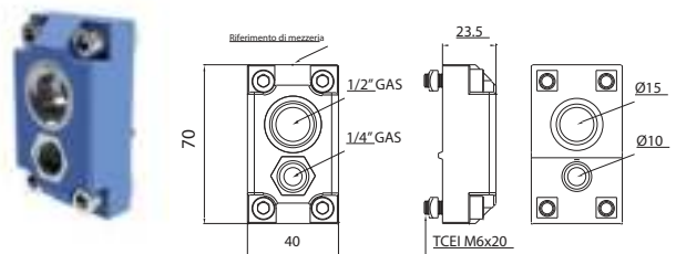
M231-012014 Toma frontal doble Ø25 1/2" - Ø16 1/4"
