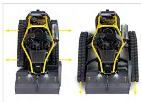
SISTEMA PATENTADO DE ELEVACIÓN con variación del centro de gravedad de la máquina
